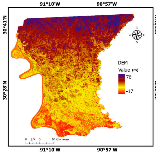
(a) DEM
