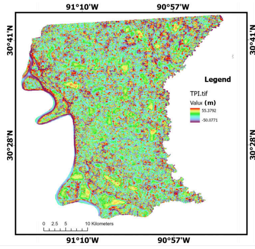
(d) TPI
