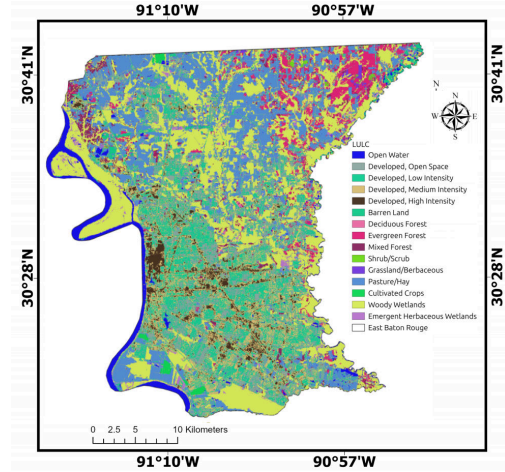
(h) LULC
