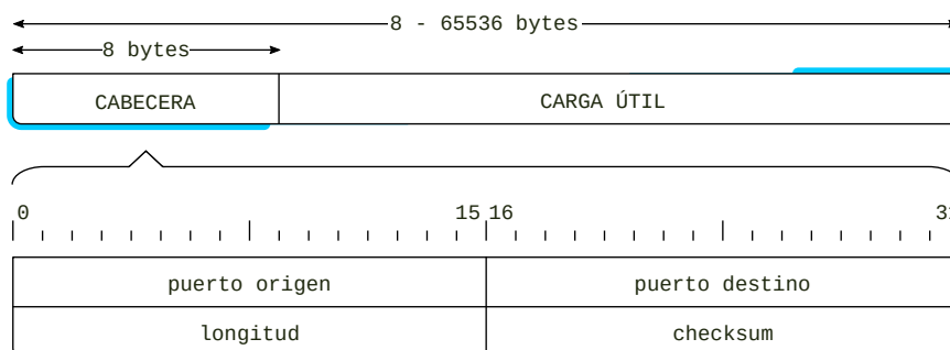
FIGURA 5.11: Formato del datagrama UDP
