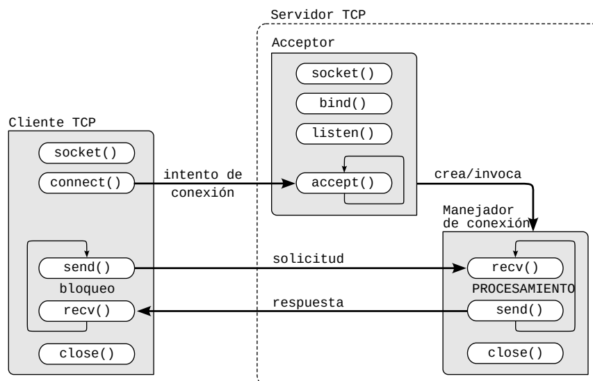
FIGURA 6.3: Diagrama de interacción de un cliente y un servidor TCP
