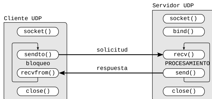
FIGURA 6.2: Diagrama de interacción de un cliente y un servidor UDP
