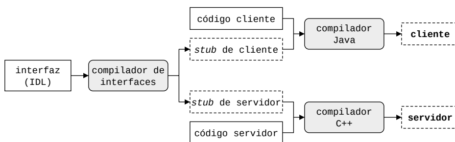
FIGURA 23.1: Generación de stubs y ejecutables a partir de la interfaz (en discontinua los archivos generados)
