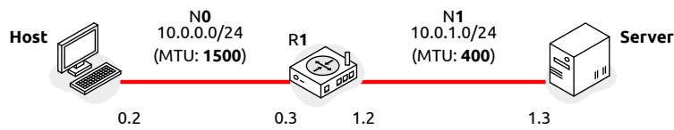
FIGURA 8.13: Topología del laboratorio de la fragmentación /lab-frag
