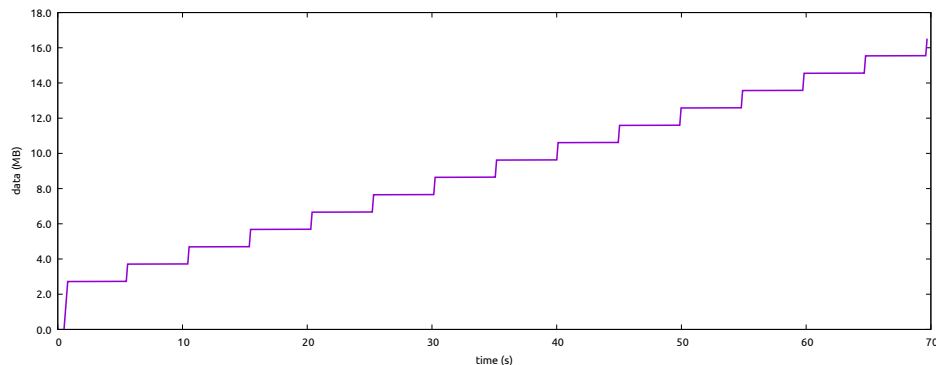
FIGURA 17.3: Datos enviados por el emisor
