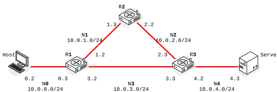
FIGURA 9.7: Topología Delta-1 con direccionamiento
