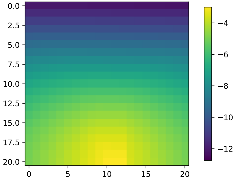
Energy (VQE)
