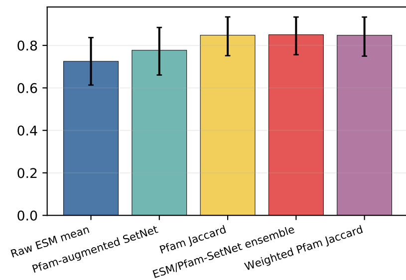
MAP
