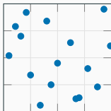
Latin hypercube
