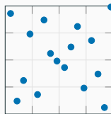
Sobol
