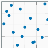
Latin hypercube
