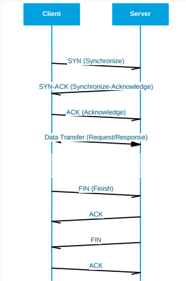
Handshake de 3 vias TCP
