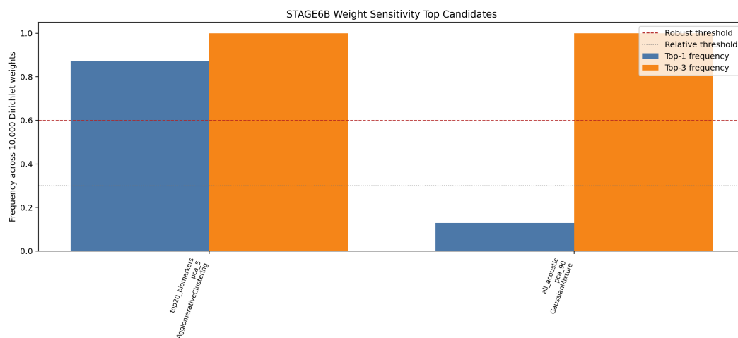
图 13 第 6b 阶段权重敏感性主要候选
