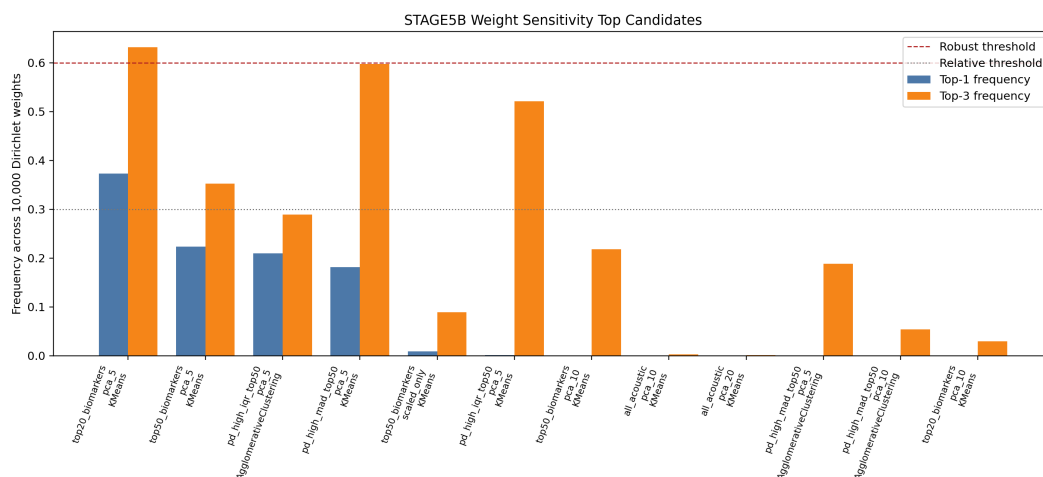
图 12 第 5b 阶段权重敏感性主要候选
