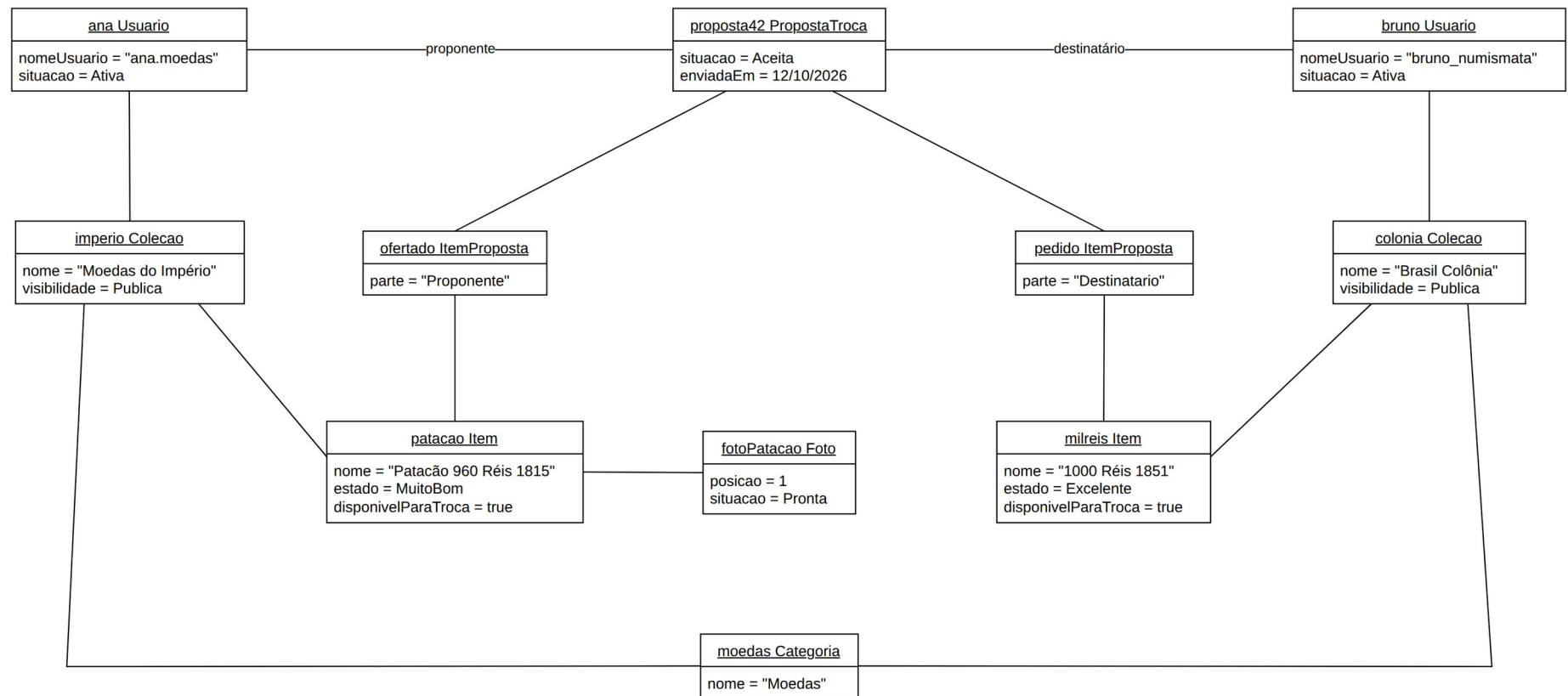
Figura 10. Diagrama de objetos de uma troca aceita
