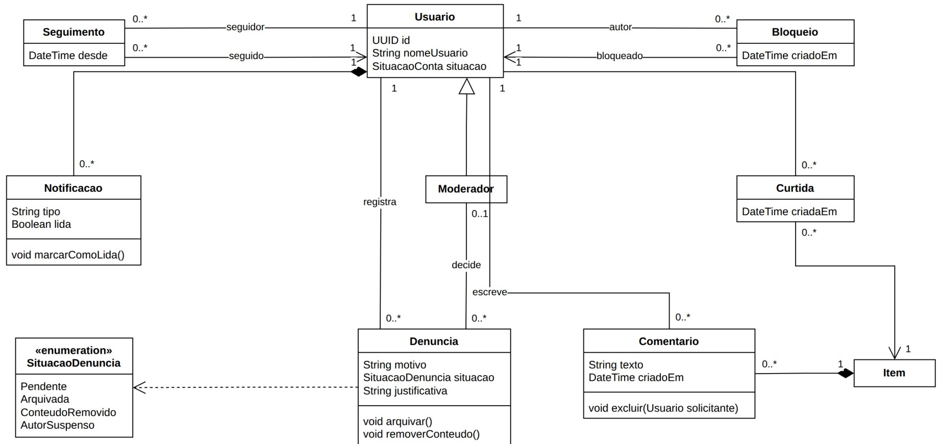
Figura 4. Diagrama de classes de social e moderação
