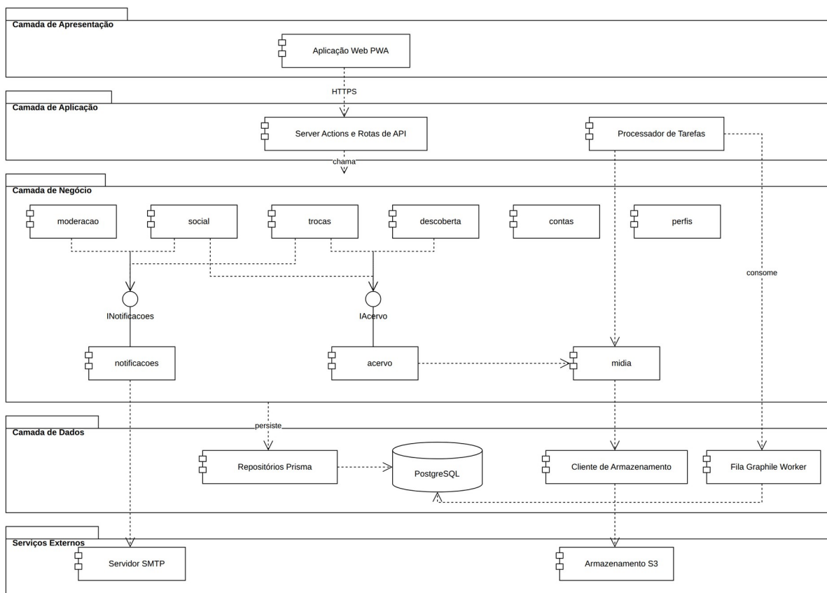
Figura 9. Diagrama de componentes do Collection Social
