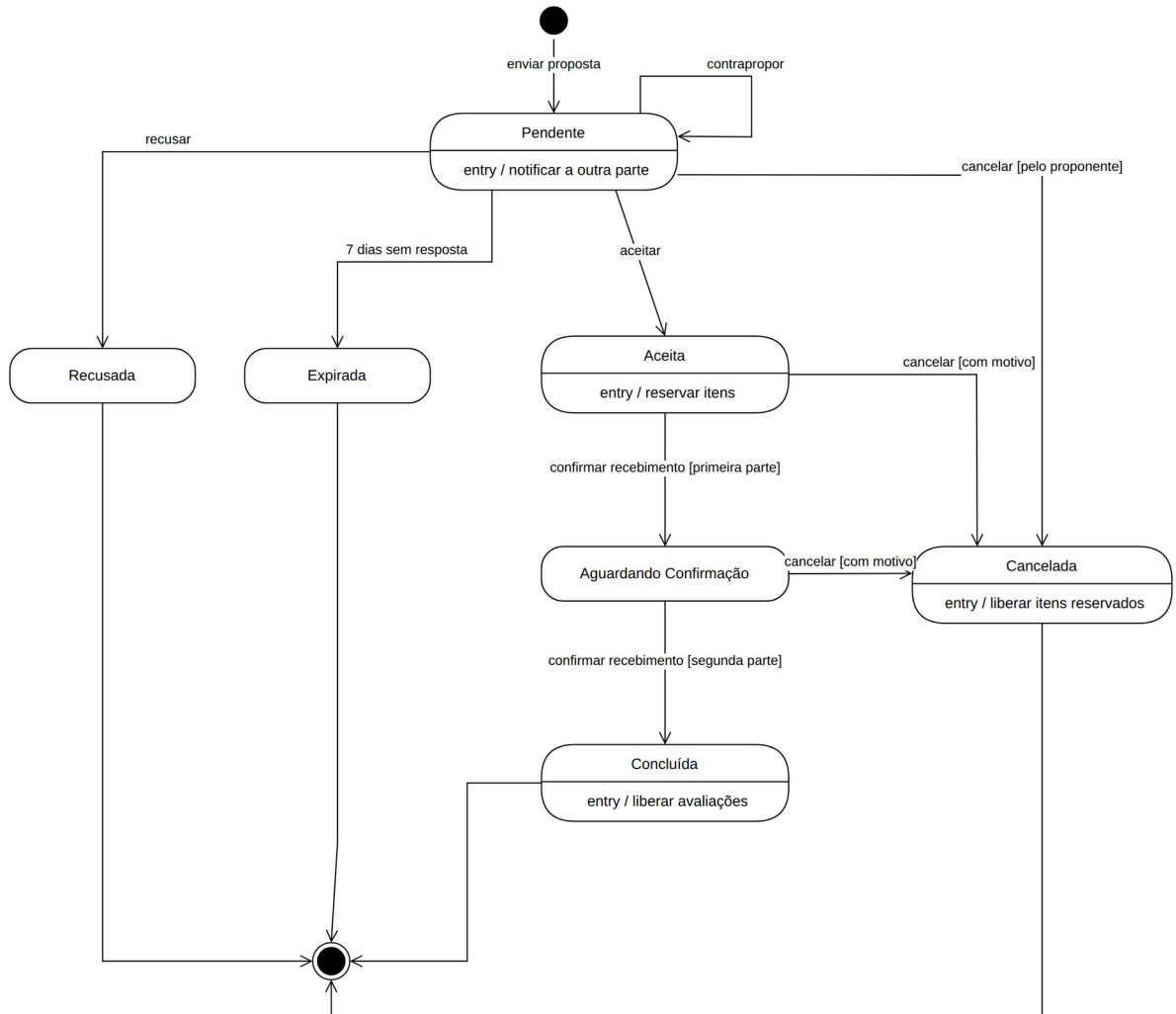
Figura 8. Diagrama de máquina de estados da proposta de troca
