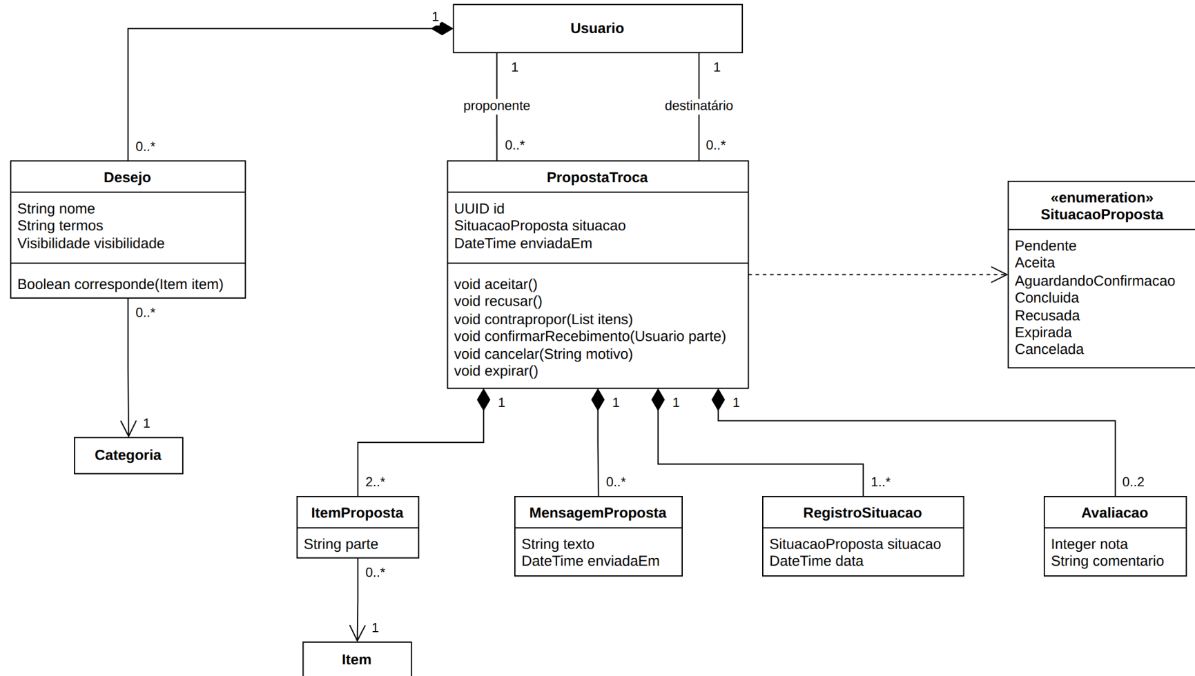
Figura 5. Diagrama de classes de trocas
