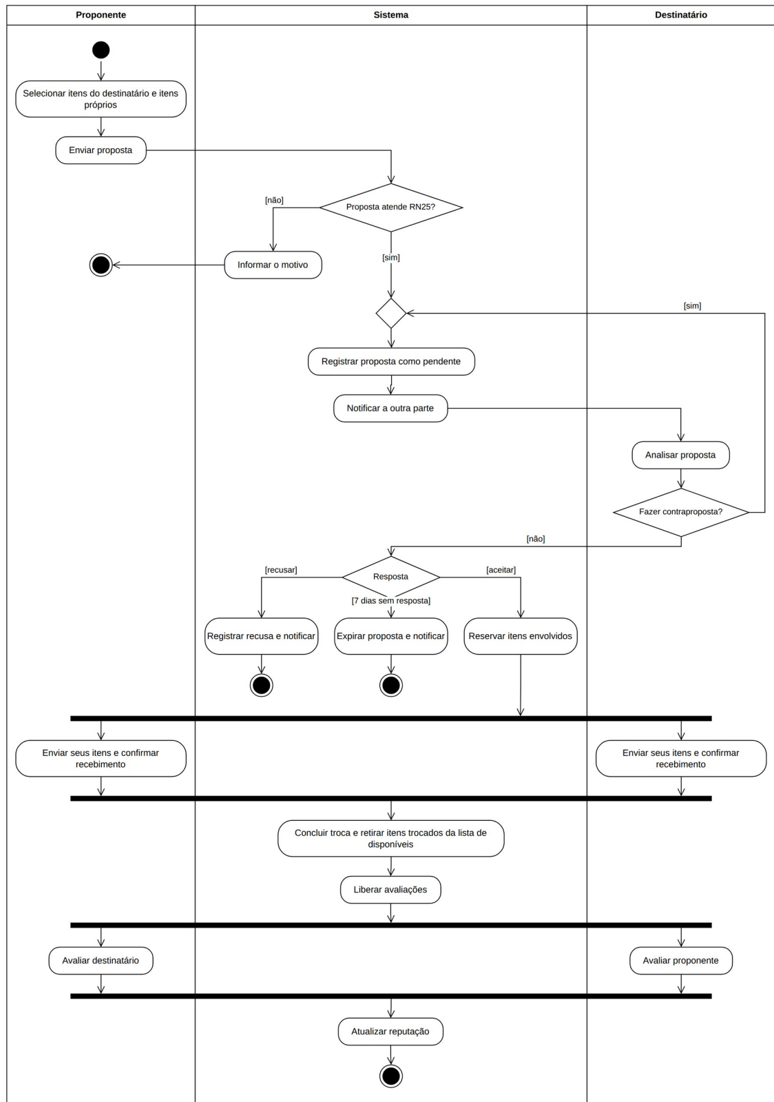
Figura 6. Diagrama de atividades do processo de troca
