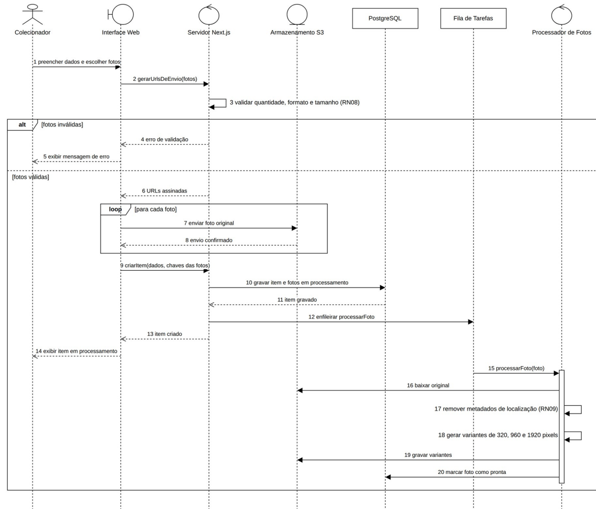
Figura 7. Diagrama de sequência do cadastro de item com fotos
