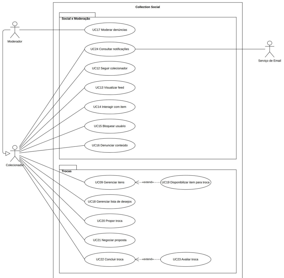
Figura 2. Diagrama de casos de uso de social, moderação e trocas
