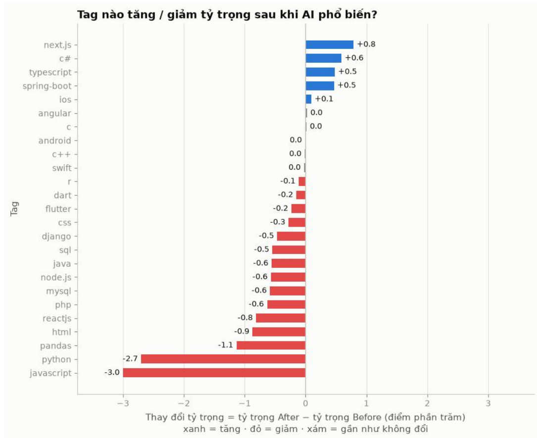
Hình 6. Thay đổi tỷ trọng của 25 tag công nghệ
