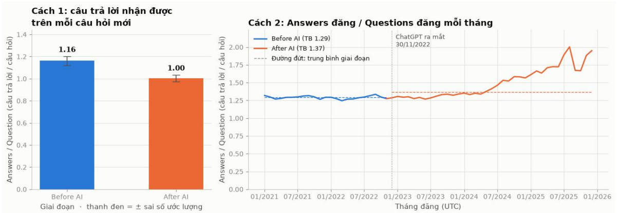
Hình 4. Số câu trả lời trên mỗi câu hỏi theo hai cách tính
