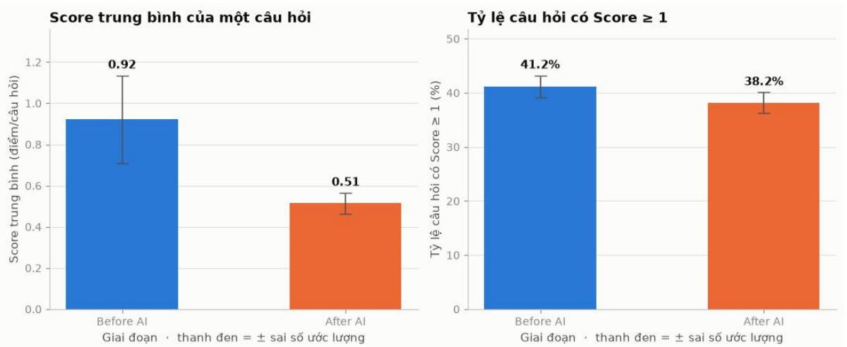
Hình 5. Score trung bình và tỷ lệ câu hỏi có Score dương
