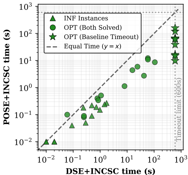
POSE+INCSC vs DSE+INCSC
