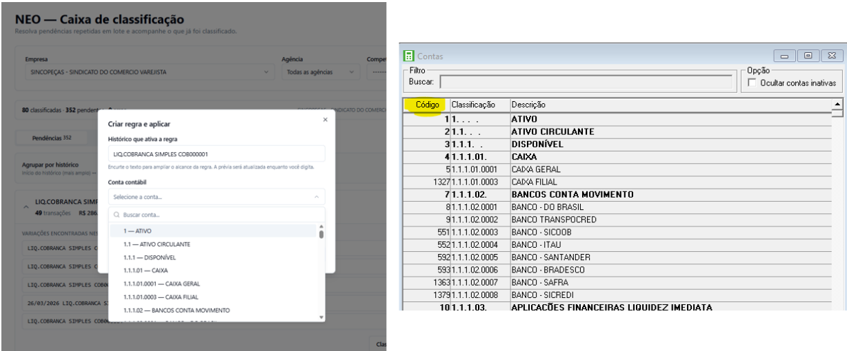
Exemplo do campo atual de seleção de conta e referência do cadastro que apresenta o código da conta.
