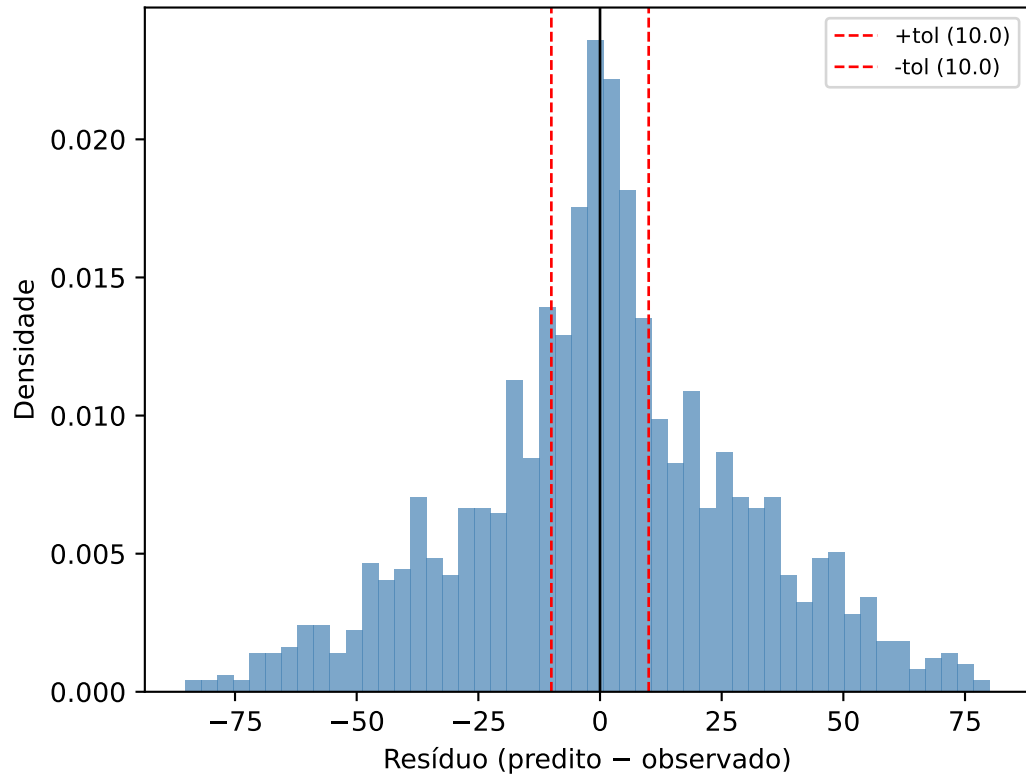
Resíduos | 35.9% dentro da tolerância
