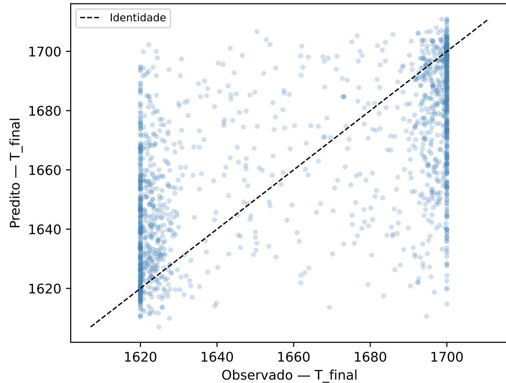
Config A (brutos) | SVR | MAE=21.8576
