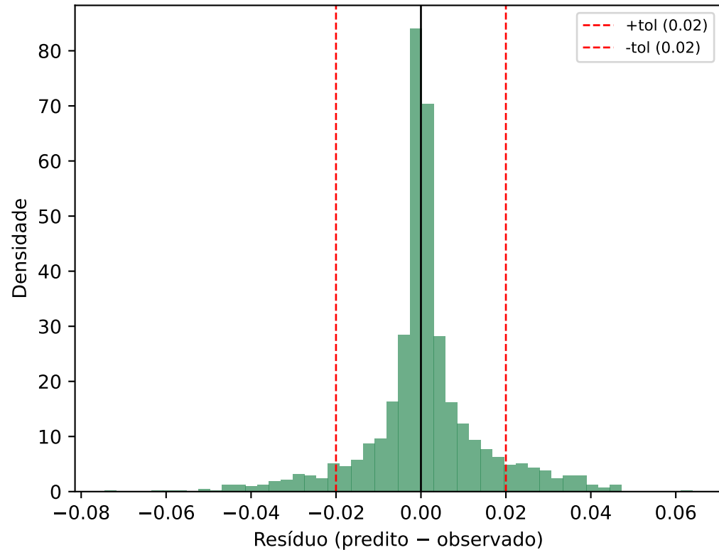
Resíduos | 85.9% dentro da tolerância
