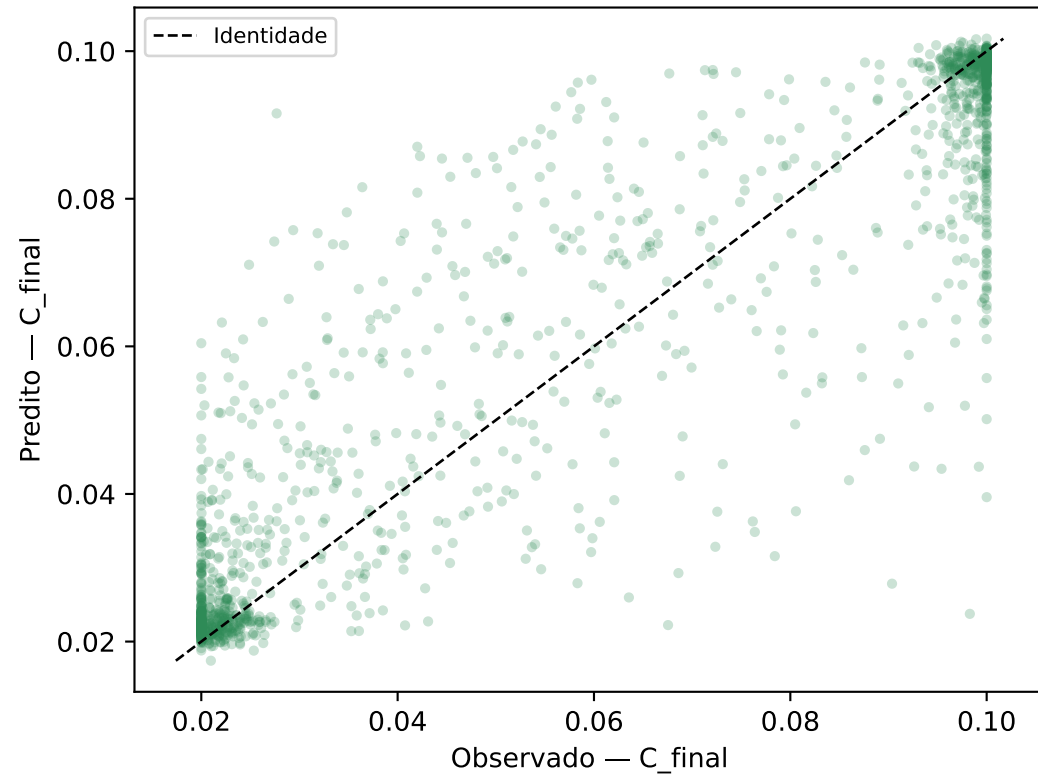
Config C (físicos) | CATBOOST | MAE=0.0086
