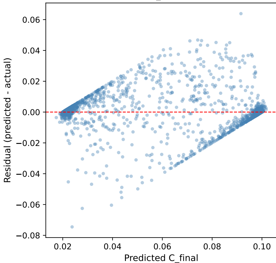
CatBoost — C_final (Config C)
