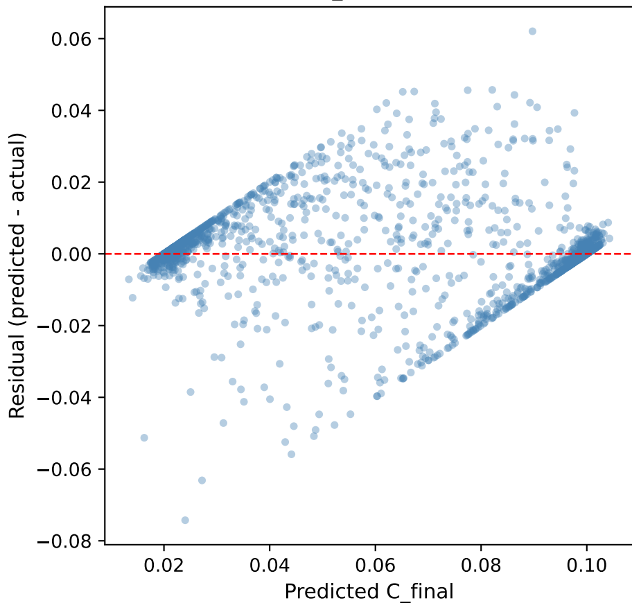
MLP — C_final (Config C)
