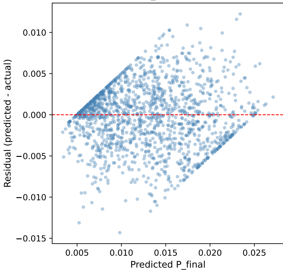
MLP — P_final (Config C)
