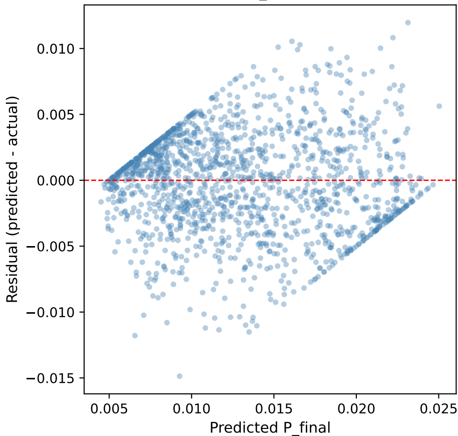
XGBoost — P_final (Config C)
