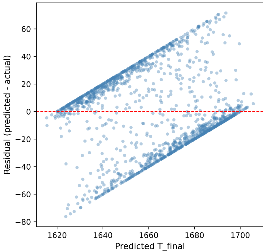
XGBoost — T_final (Config C)
