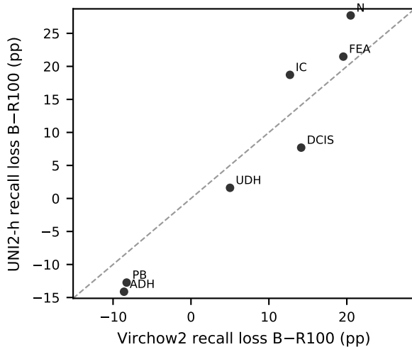
BRACS
