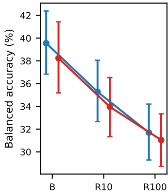
BRACS
