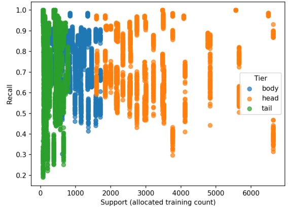
(d) TCGA-UT
