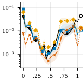
Gemma-3-1B-PT
