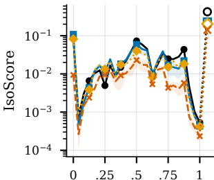
EmbeddingGemma-300M
