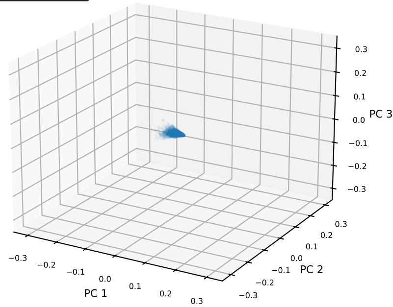
Layer 27 (N-1)
