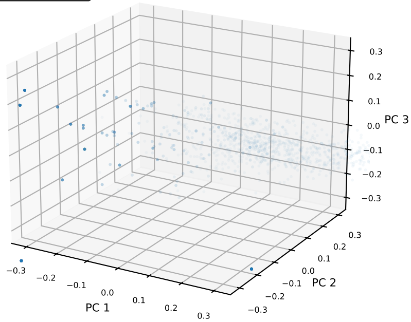
Layer 17
