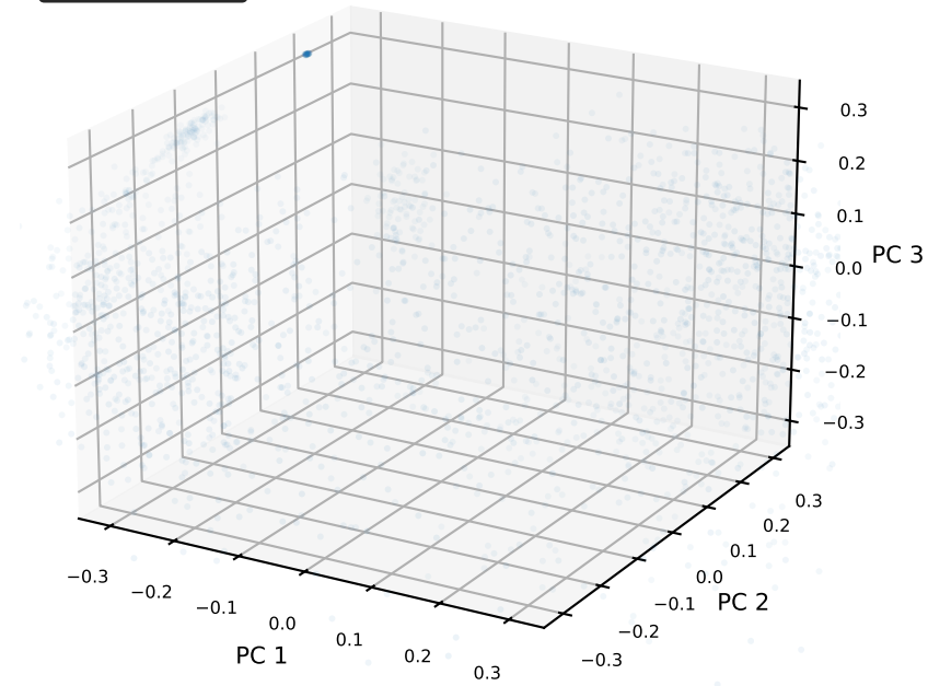
Layer 23 (N-1)
