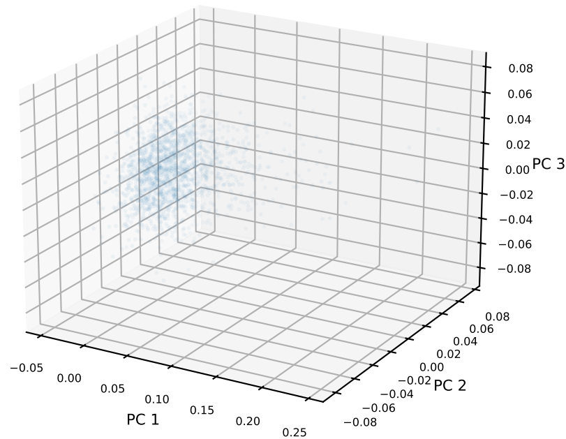
Layer 20
