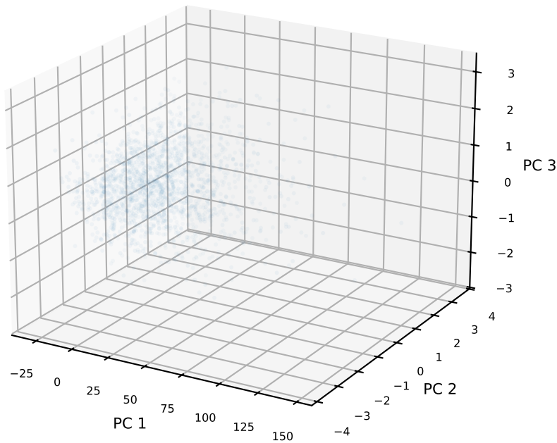
Layer 27 (N-1)
