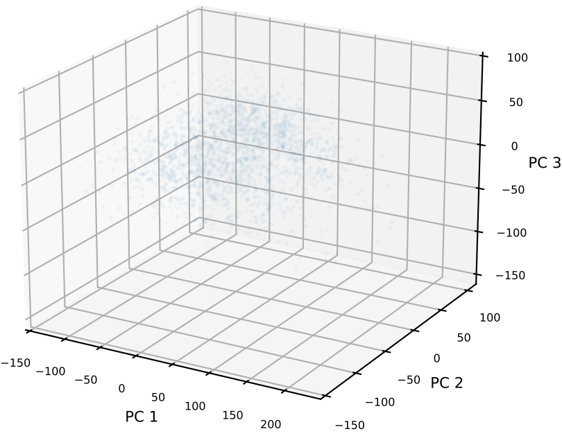
Layer 23 (N-1)
