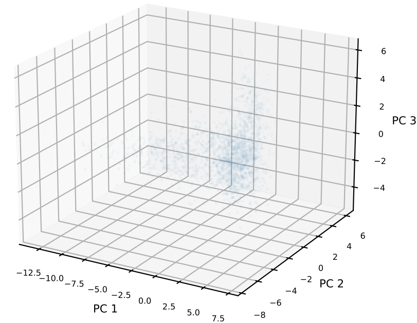
Layer 17
