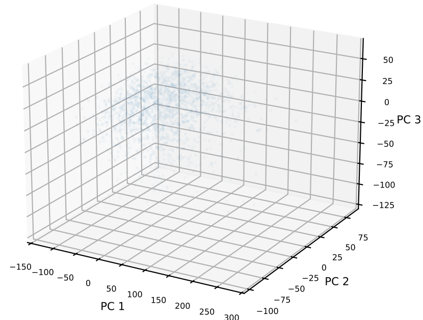
Layer 23 (N-1)
