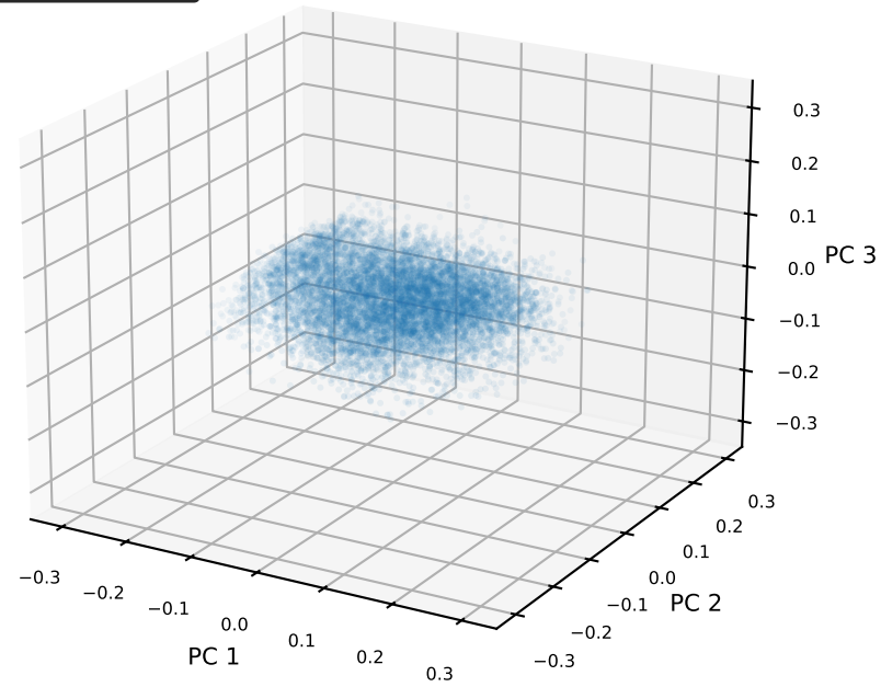
Layer 27 (N-1)
