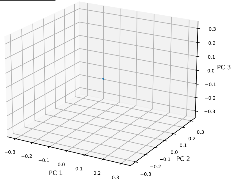
Layer 20
