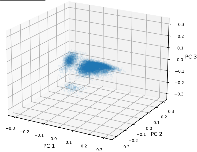
Layer 27 (N-1)
