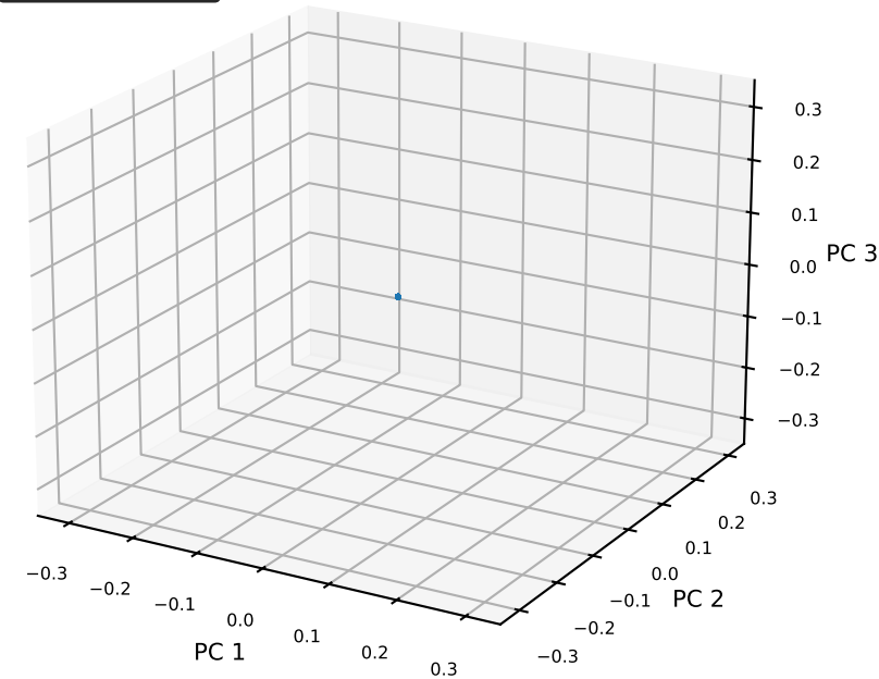
Layer 20
