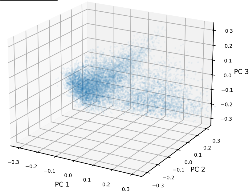
Layer 17
