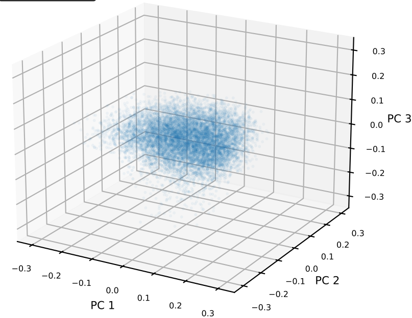
Layer 23 (N-1)
