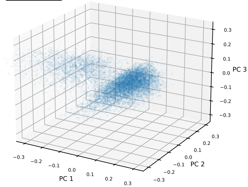
Layer 17
