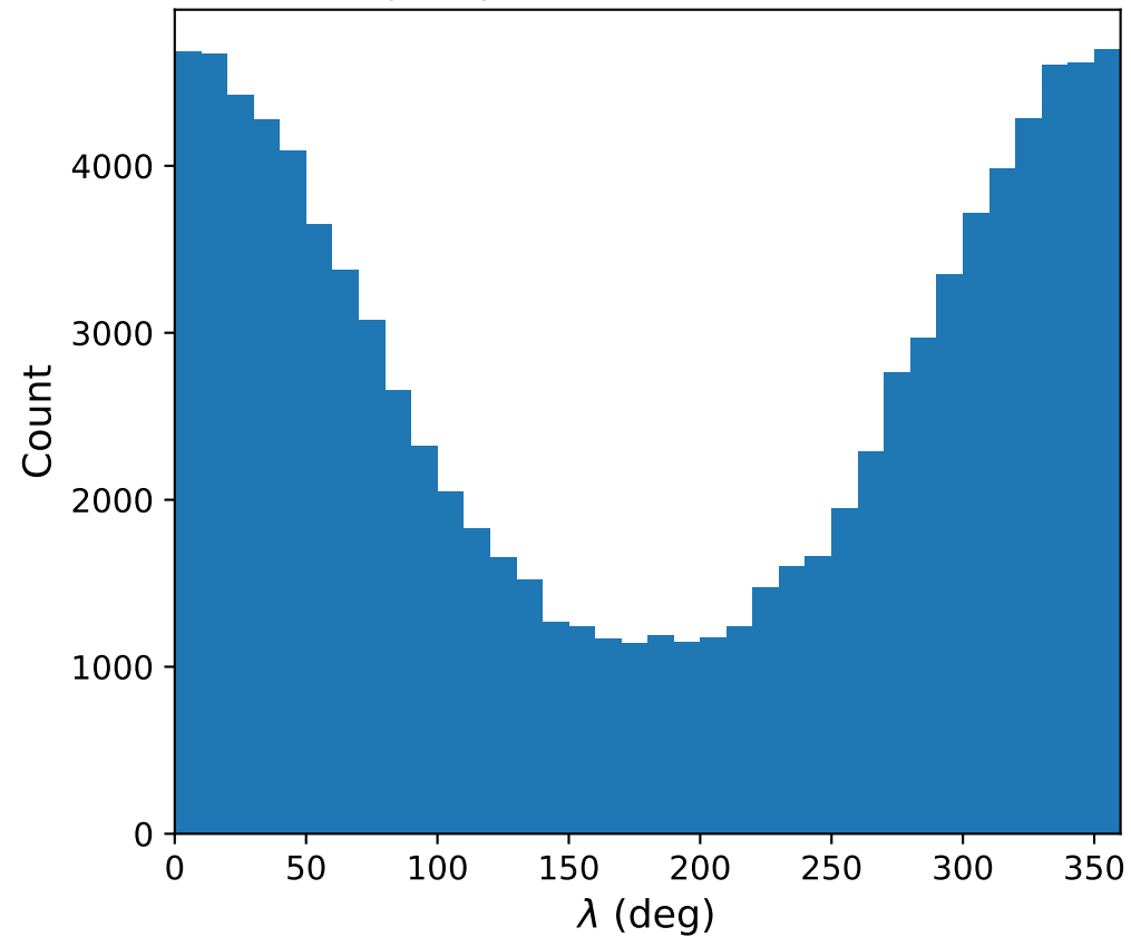
MBA ( |\beta| < 3.0^\circ ): longitude histogram
