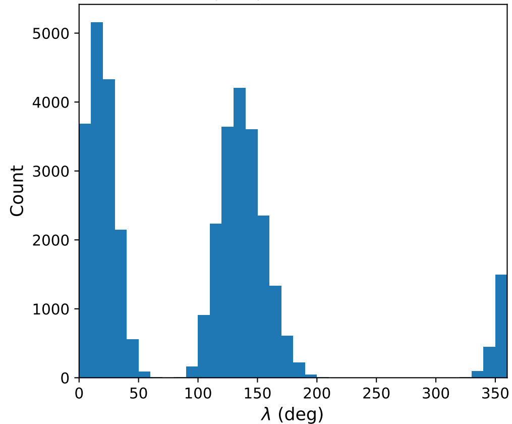
Jupiter Trojans ( |\beta| < 3.0^\circ ): longitude histogram
