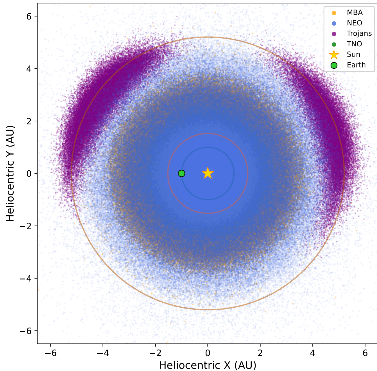
Inner solar system (0-6.5 AU)
