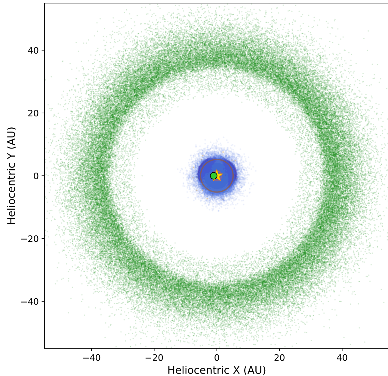
Full solar system incl. TNOs (0-55 AU)
