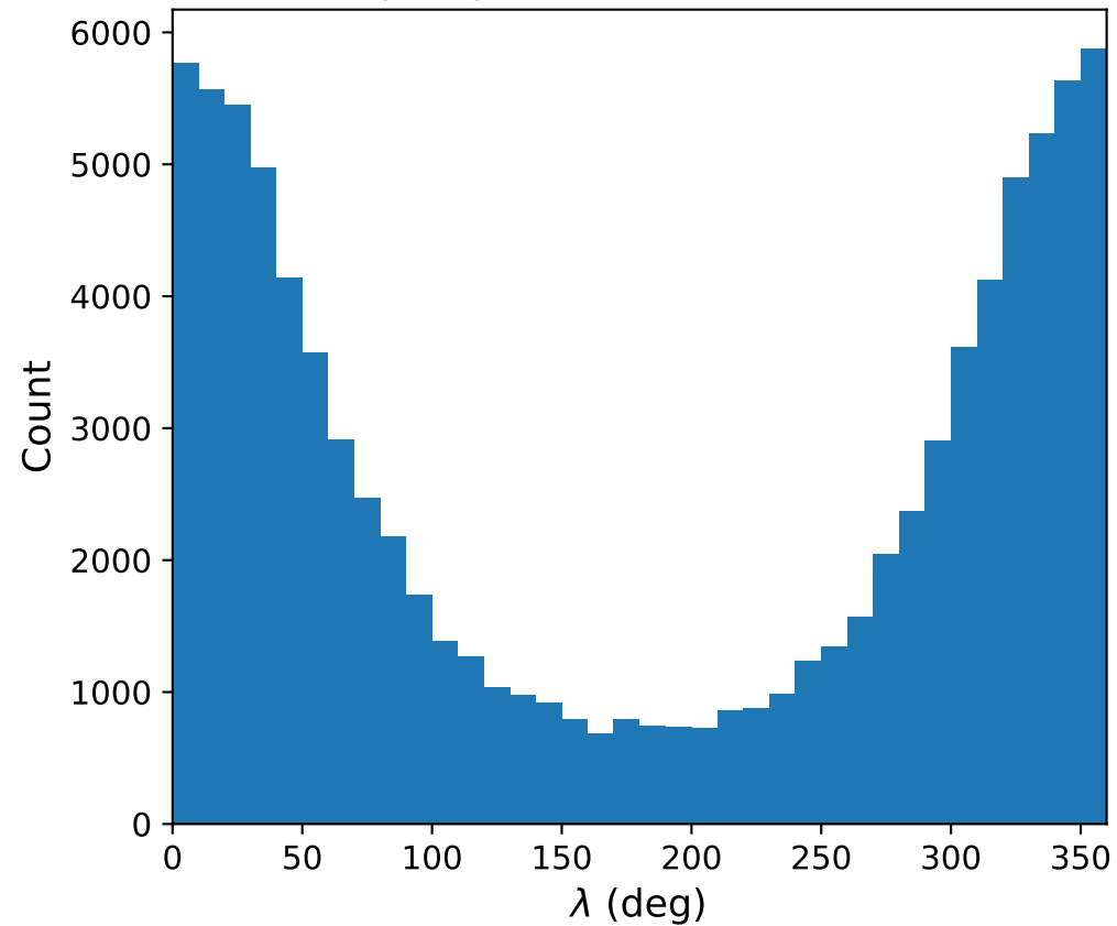
NEO ( |\beta| < 3.0^\circ ): longitude histogram
