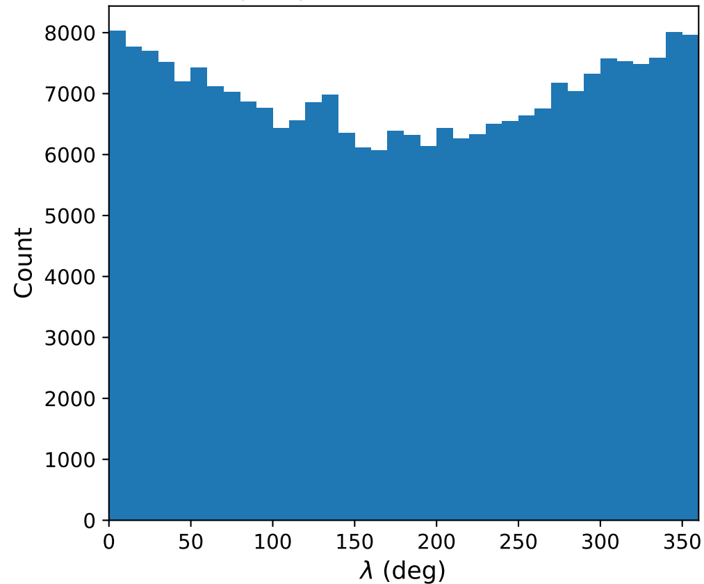
TNO ( |\beta| < 3.0^\circ ): longitude histogram
