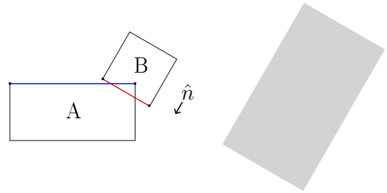
Figura 15 – Aresta de referência em vermelho e aresta incidente em azul.
