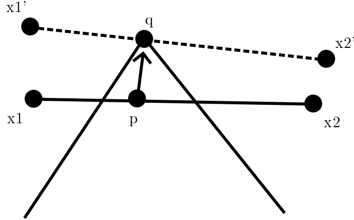
Figura 13 – Processo de separação caso colisão vértice-aresta. Correção das posição para configuração válida. Perceba que, como p está mais próximo de x_1 , esse vértice é movido mais.
