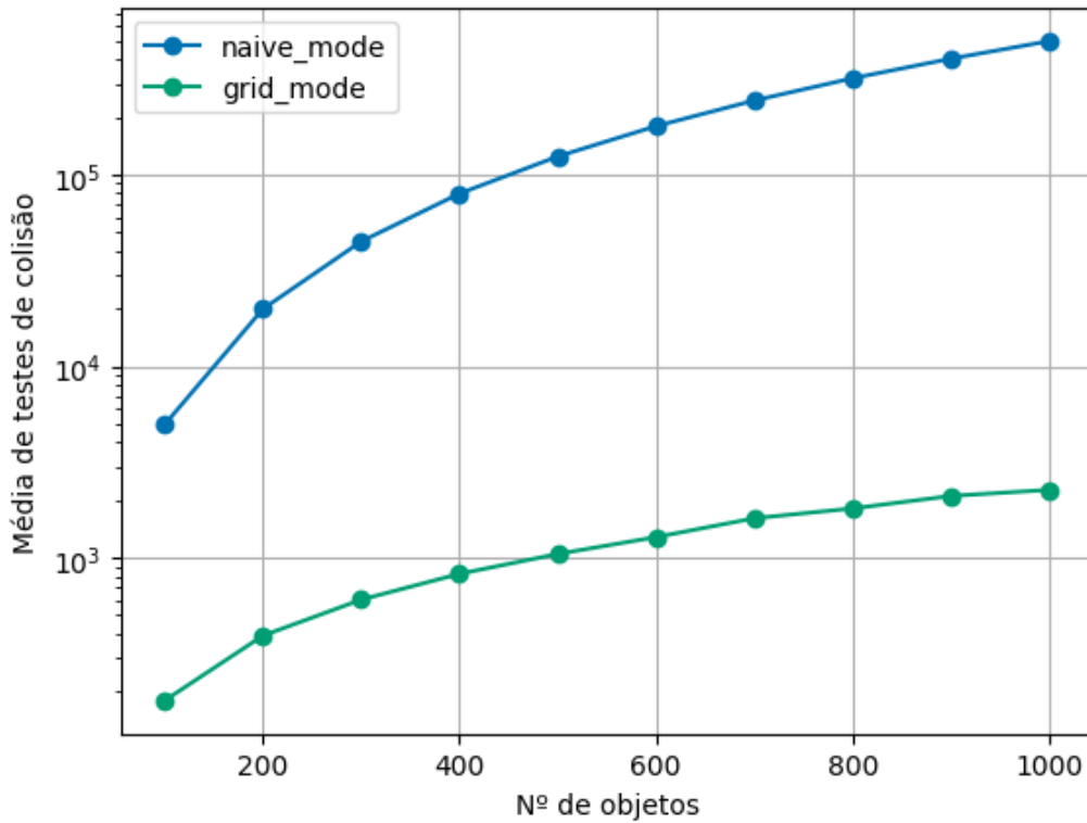
Figura 23 – Número médio de testes de colisão em função do número de objetos, com e sem utilização de grade uniforme no filtragem, na nossa implementação. Fonte: Autor.
