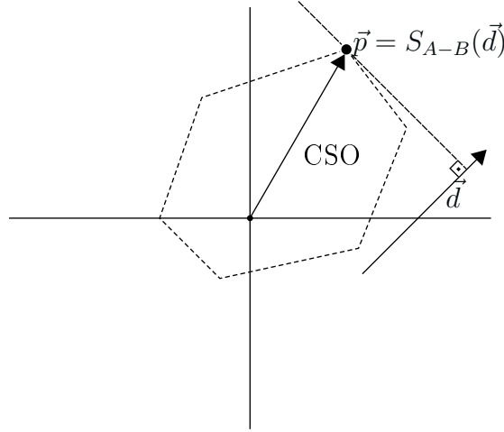
Figura 7 – A função suporte na forma implícita A - B ao longo da direção \vec{d} . Fonte: Autor.
