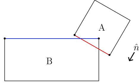
Figura 14 – Aresta de referência em vermelho e aresta incidente em azul. Fonte: Adaptado de (Newcastle University, 2017).
