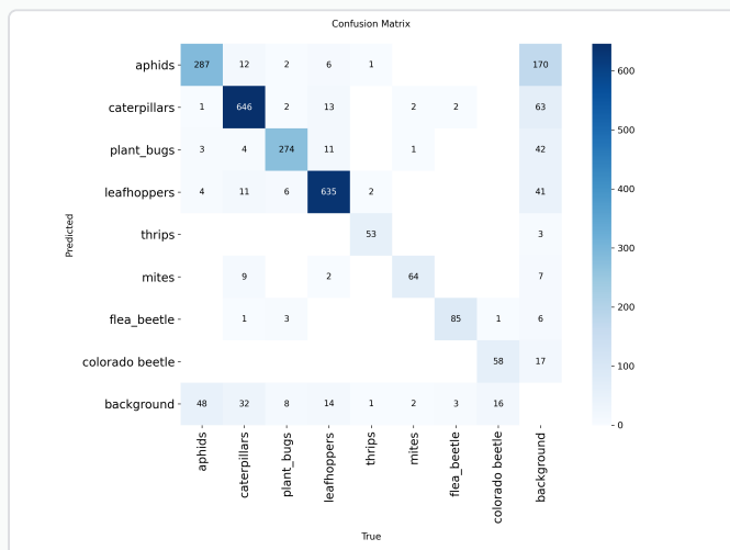
Figure 2 : Matrice de Confusion (Valeurs absolues)
