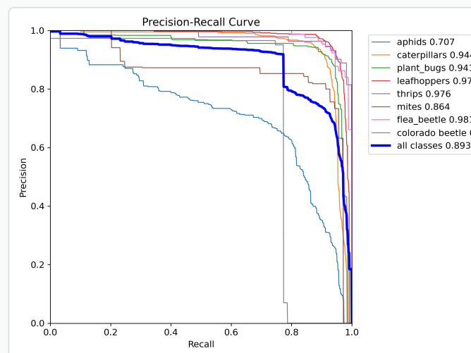
Figure 5 : Courbe Précision-Rappel (AUC)
