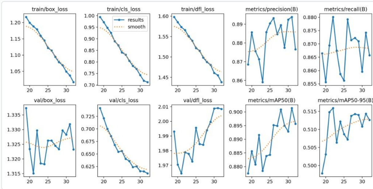
Figure 1 : Évolution des pertes et des métriques d'entraînement par époque
