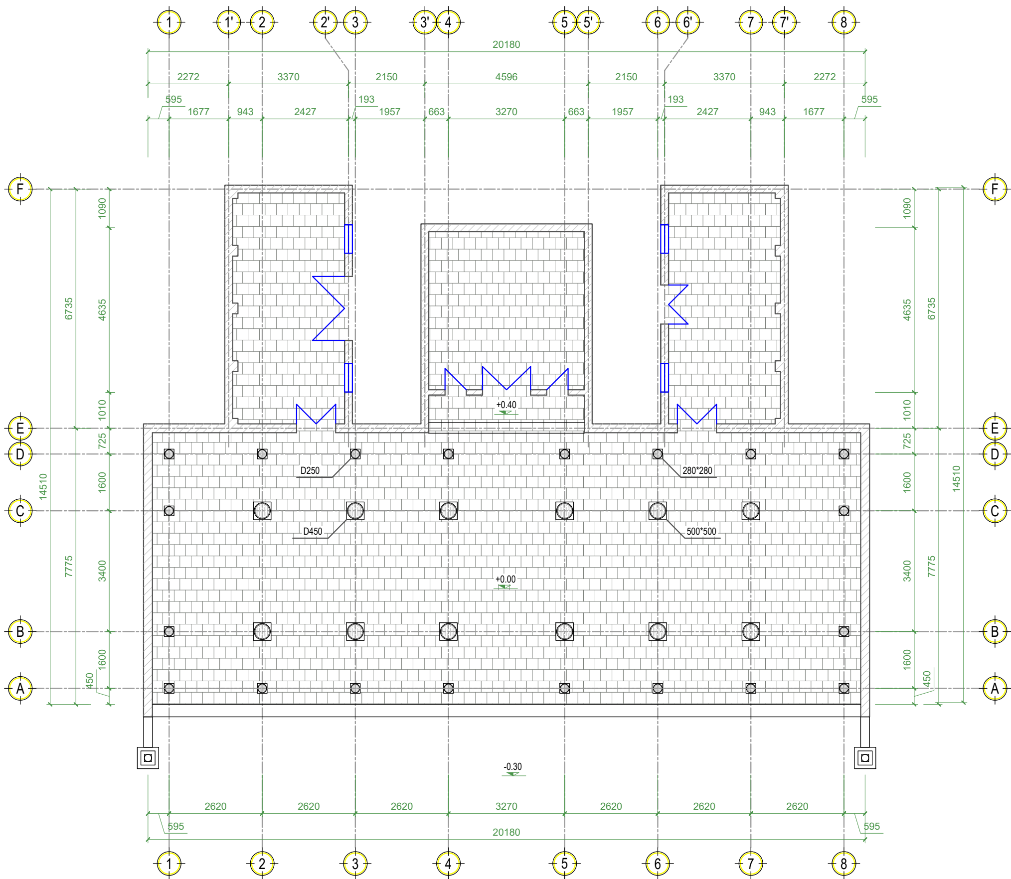
MẶT BẰNG
