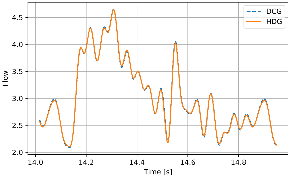
ulnar_L Flow
