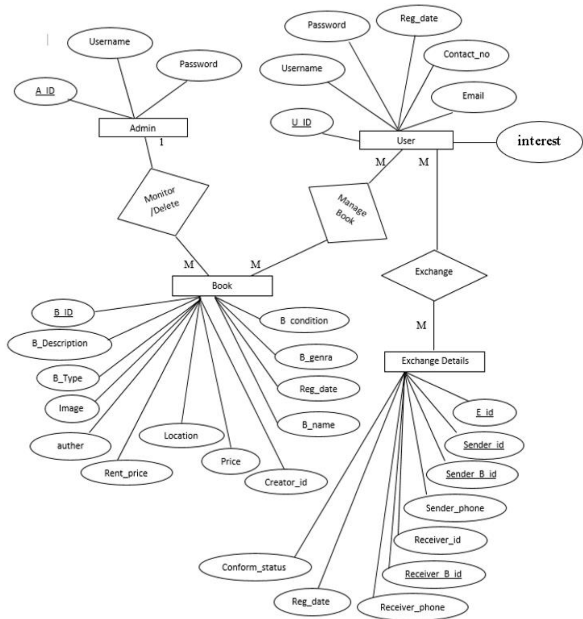
Figure 2: ER diagram
