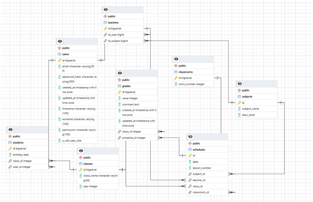
Рисунок 1.6.10 – ERD диаграмма
