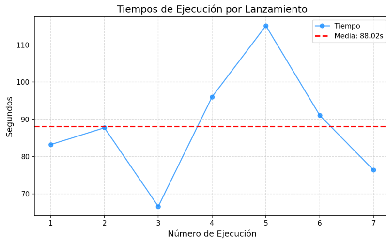
Figure 8: Distribución de tiempos de ejecución - Modelo B.
