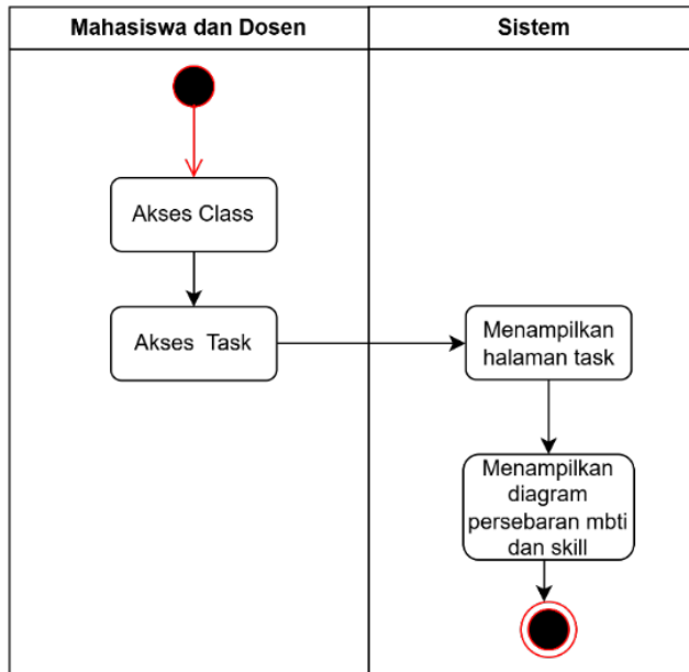
Gambar 3.7 Activity Diagram Melihat Persebaran MBTI, Keahlian, Preferensi, dan Jenis Kelamin Mahasiswa
